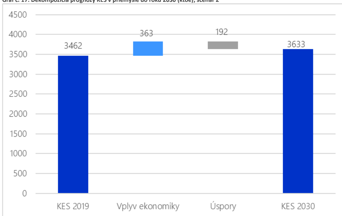
Graf č. 17: Dekompozícia prognózy KES v priemysle do roku 2030 (ktce), scenár 2
