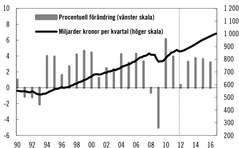
Diagram 1 Svensk BNP
